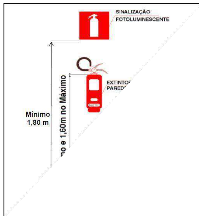
Figura 40: Detalhamento para instalação de extintor de incêndio.
