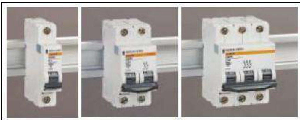
Figura 23: Disjuntores termomagnéticos norma DIN. Ref.: Siemens ou similar.
