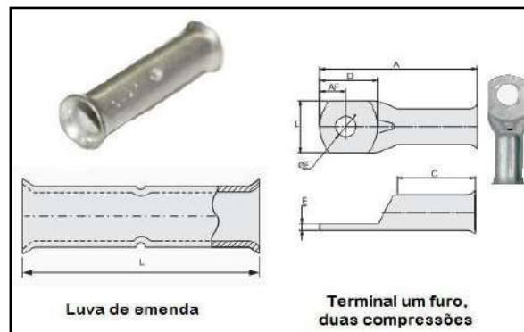
Figura 35: Luva e terminal a compressão de cobre estanhado
