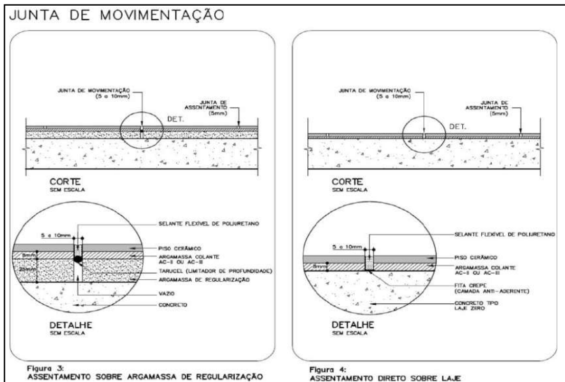
Figura 19: Junta de Movimentação
