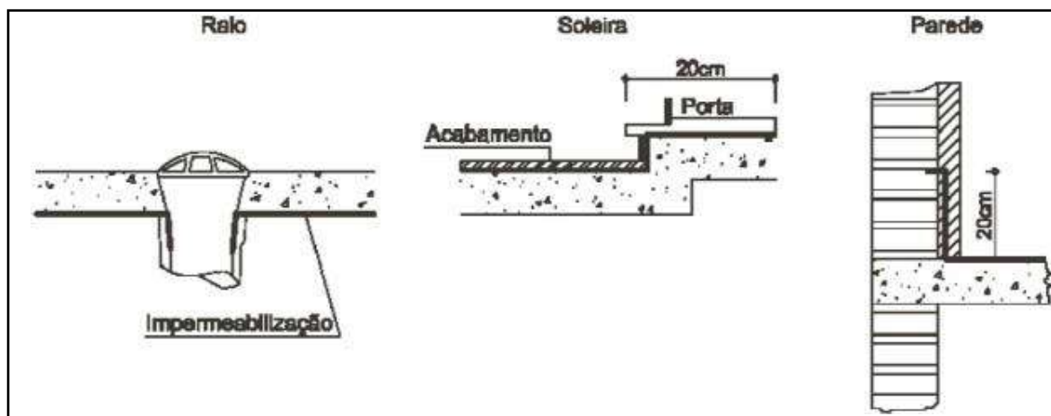
Figura 20: Impermeabilização com Vedapren (06 demãos)
