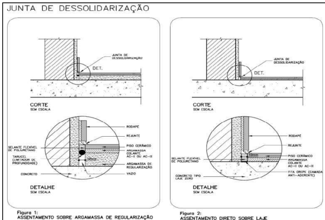
Figura 18: Junta de Dessolidarização
