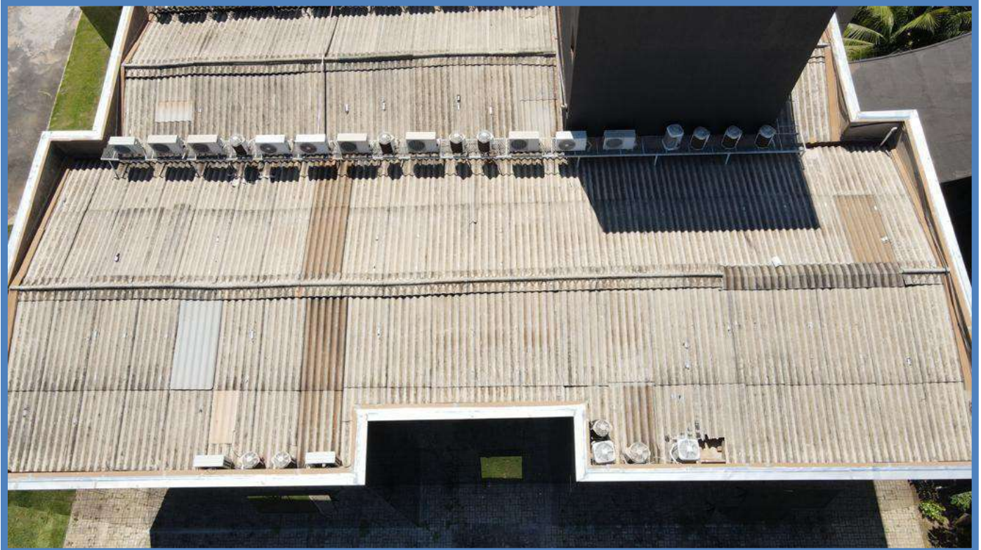
Figura 248: FOTOS AÉREAS - COBERTURA
