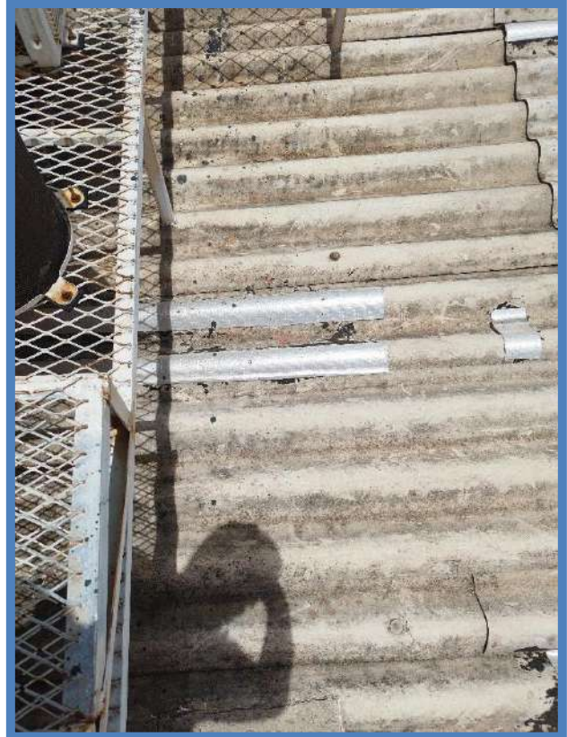
Figura 208: BLOCO B – COBERTURA
