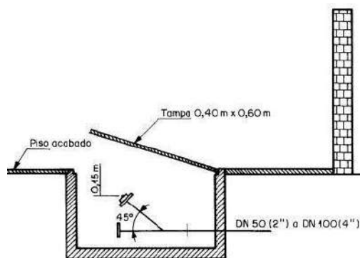
Figura 37: Dispositivo para recalque
