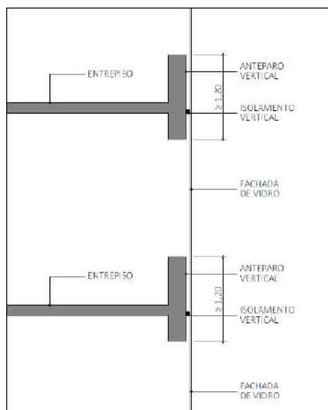
Figura 42: Modelo de compartimentação com fachada envidraçada
