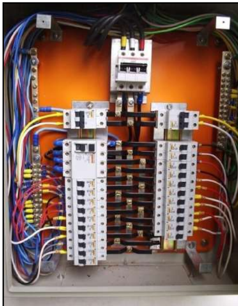
Figura 22: Vista interna do Quadro de Disjuntores
